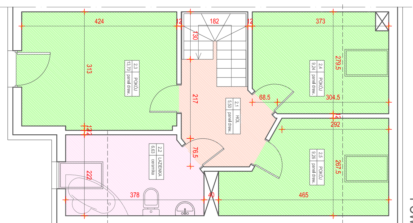
ZESTAWIENIE POWIERZCHNI UŻYTKOWEJ NETTO (po podłodze) PIĘTRA
